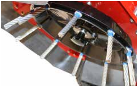
Patentierter Werkzeugteller mit werkzeuglosem Schnellwechselsystem zum Borstenwechsel (ab TW 50)
