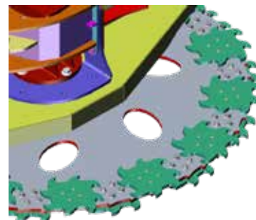
Mähscheibe Interpiquet High Cut mit auswechselbaren Messern
